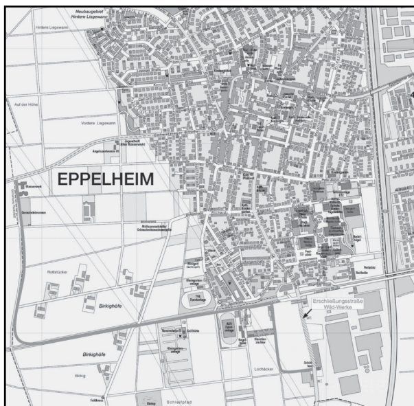
Planvorschlag Umgehungsstraße
